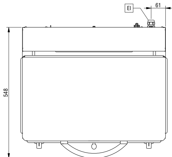
Planta
